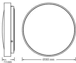
CEILING LUXO 24W
