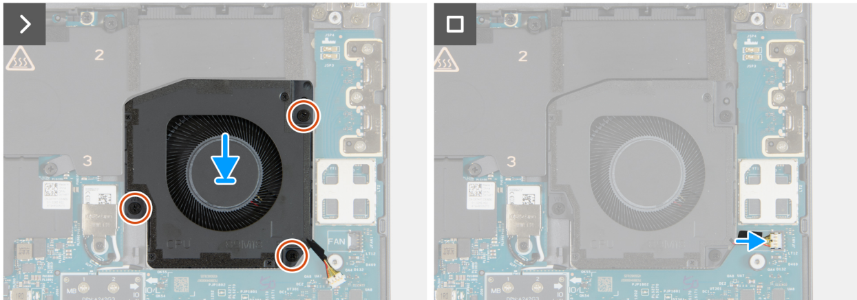
Figure 28. Installing the left fan
