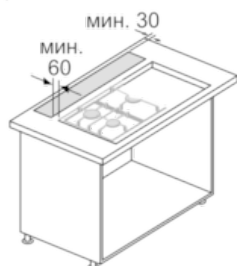
Комбинация с газов плот 75 см
