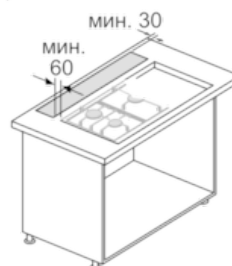
Комбинация с газов плот 90 см
