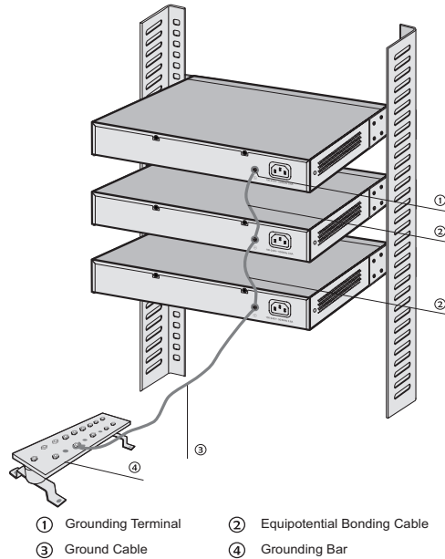
Figure 3-3 Equipotential Bonding
